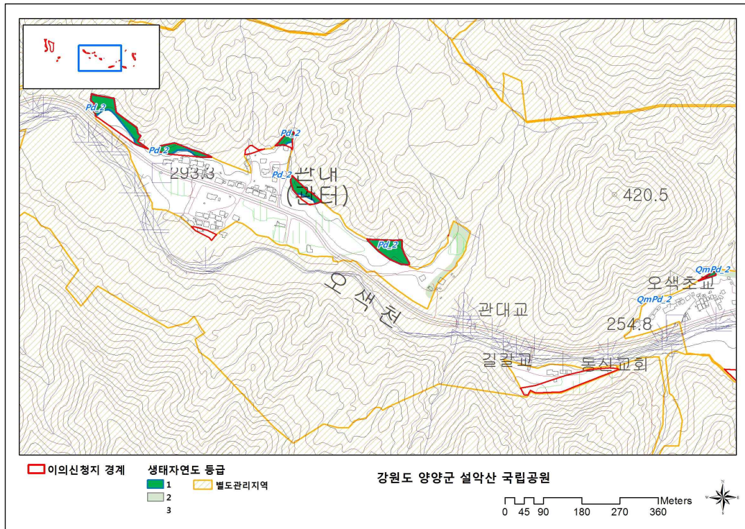
<설악(388144) 도엽 수정·보완 도면-2>
